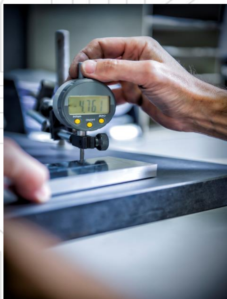
Pièce de précision en Aluminium usinée dans la masse
